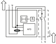
5SM6011-1
